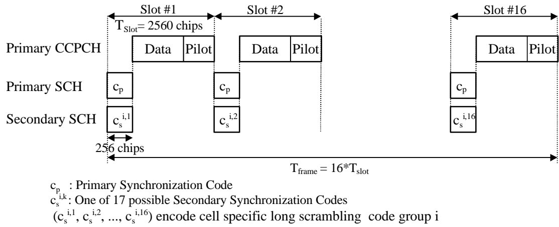
Figure 1545: Structure of Synchronisation Channel (SCH).
