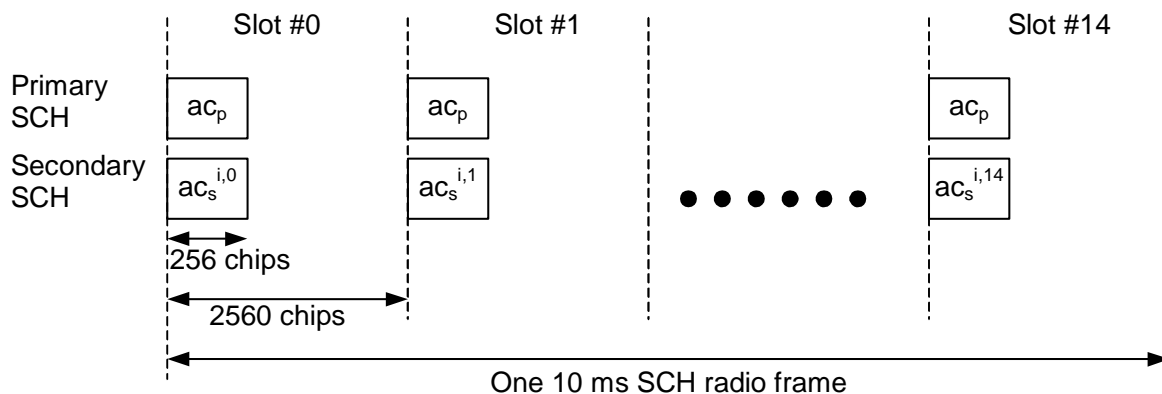
Figure 1820: Structure of Synchronisation Channel (SCH)
