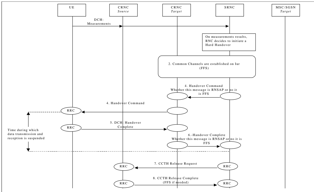
Hard Handover via Iur
